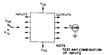
Fig. 14 - Input voltage test circuit.
