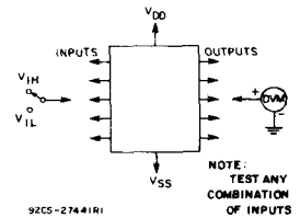
Fig. 12 — Input-voltage test circuit.
