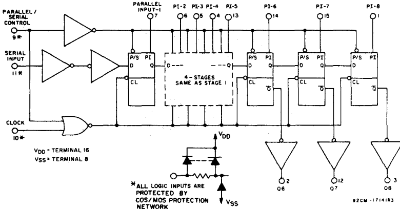
Fig. 5 - Logic diagram.
