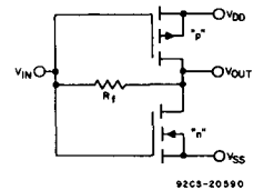
Fig. 5 - COS/MOS amplifier.
