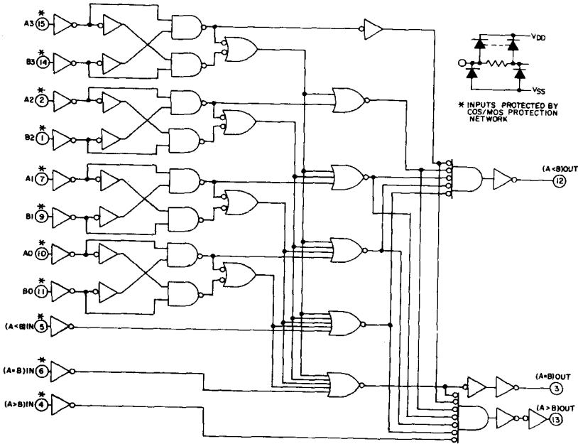
Fig. 4 - Logic diagram.
