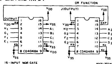
16- INPUT NOR GATE J = A1 + B1 + C1 + D1 + E1 + F1 + G1 + H1 + A2 + B2 + C2 + D2 + E2 + F2 + G2 + H2 Fig. 5 - 16-input NOR gate.
