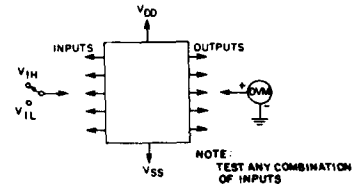
Fig. 12— Input voltage test circuit.
