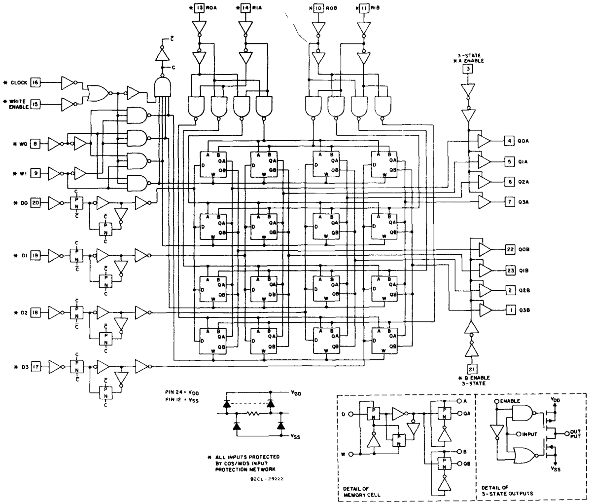
Fig. 2 - Logic diagram.
