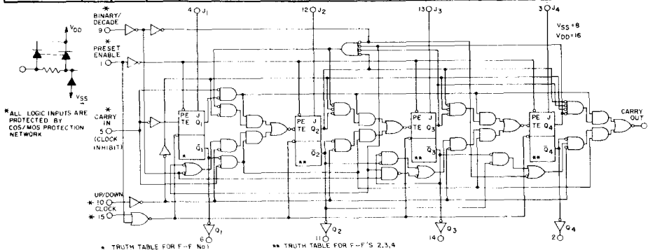
Fig. 11—Logic diagram.
